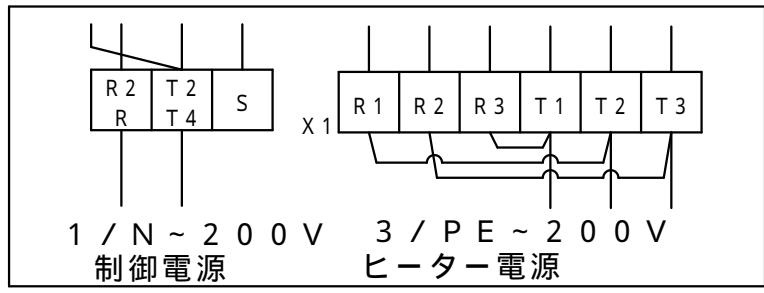
三相結線の場合
