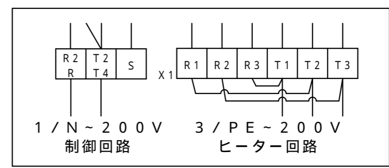
三相結線の場合
